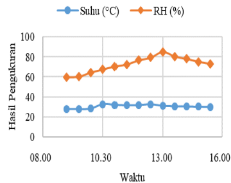
Gambar 14. Grafik hasil pengujian suhu dan kelembapan lingkungan
