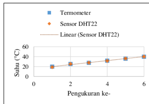
Gambar 13. Grafik hasil pengujian suhu
