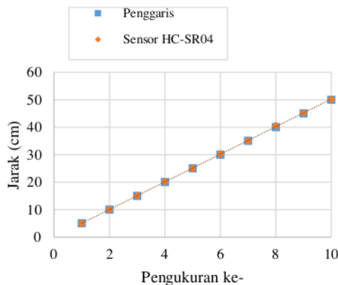
Gambar 11. Grafik hasil uji jarak
