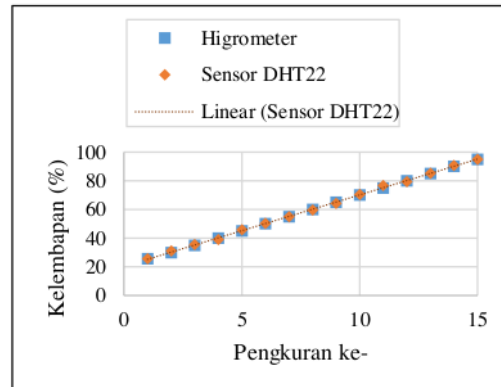
Gambar 12. Grafik hasil pengujian kelembapan
