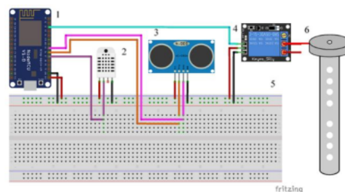
Gambar 6. Skema rangkaian elektronika
