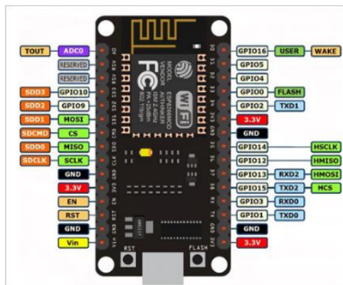
Gambar 4. NodeMCU ESP8266
