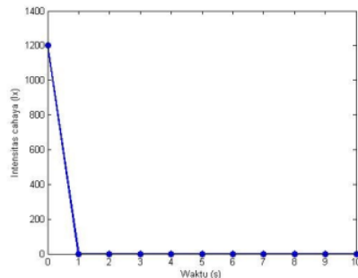
Gambar 7. Grafik pengujian sensor BH1750 ketika lampu dimatikan.
