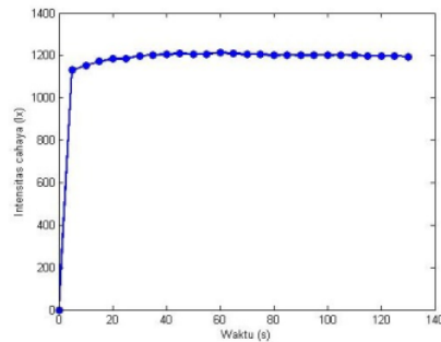
Gambar 6. Grafik pengujian sensor BH1750 ketika lampu dinyalakan.
