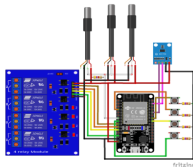
Gambar 2. Rangkaian elektronika.
