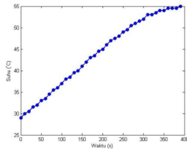
Gambar 10. Grafik pengujian sensor DS18B20 ke-2 ketika dispenser dinyalakan.
