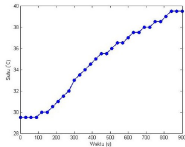
Gambar 12. Grafik pengujian sensor DS18B20 ketiga ketika rice cooker dinyalakan.
