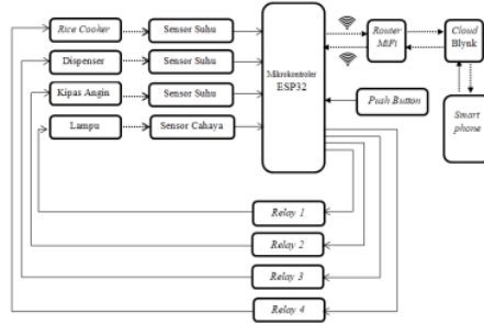
Gambar 1. Diagram blok perancangan sistem.
