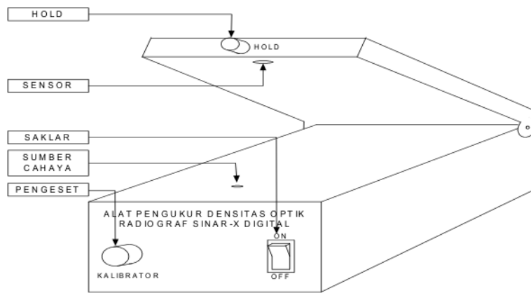
Gambar 4 Densitometer tampak dari depan
