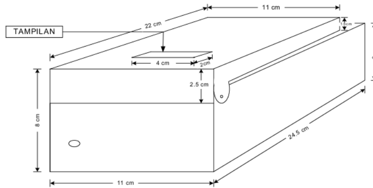
Gambar 3 Densitometer terlihat dari belakang
