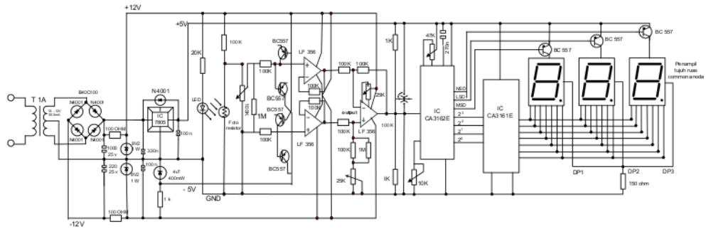
Gambar 2 Rangkaian alat densitometer
