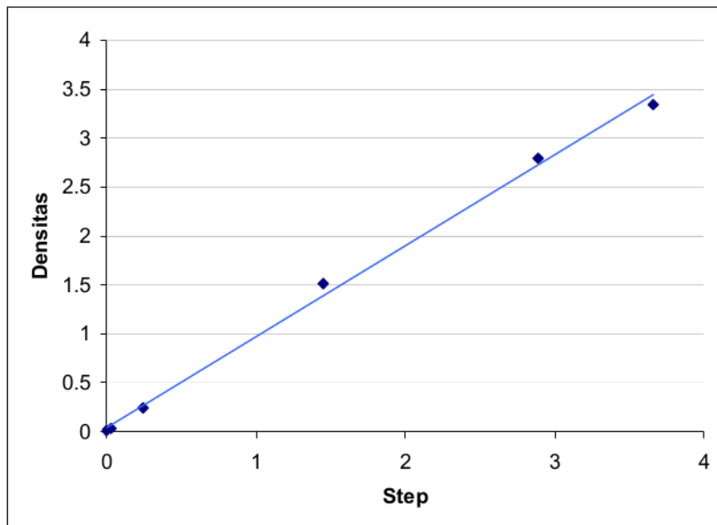
Gambar 6 Hasil kalibrasi alat menggunakan quality control
