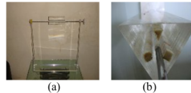
Gambar 2 (a) foto Obyek Putar dan (b) Tampang lintang Obyek Putar
