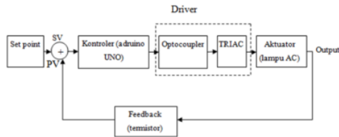
Gambar 3. Diagram blok sistem.
