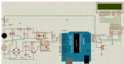
Gambar 4. Layout sistem kendali temperatur.
