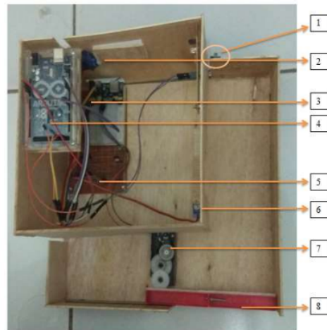
Gambar 7. Sistem Kontrol LPPJ, yang terdiri dari beberapa komponen, diantaranya: 1. Sensor LDR, 2. Motor Servo2, 3. IC L293D, 4. Arduino Mega2560, 5. Bluetooth, 6. Motor Servo2, 7. Motor DC dan gear box , dan 8. Pagar.
