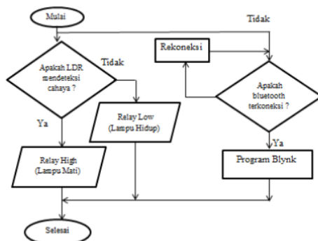
Gambar 5 . Diagram blok sistem.
