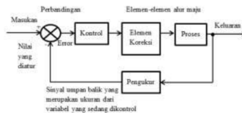
Gambar 2. Diagram blok sistem kontrol loop tertutup [4].
