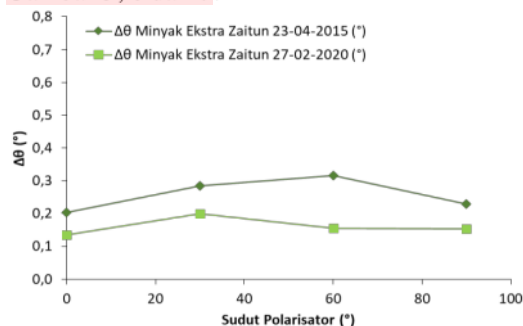
Gambar 5. Rata-rata perubahan sudut analisator digital terhadap posisi sudut polarisator menggunakan minyak zaitun.
