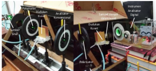
Gambar 3. Analisator Digital dalam Instrumen Polarimeter.
