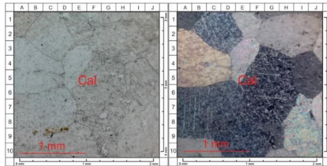
Gambar 10. Kenampakan mikroskopis batugamping kristalin dalam pengamatan nikol sejajar (kiri) dan nikol bersilang (kanan), ket: Cal = kalsit
