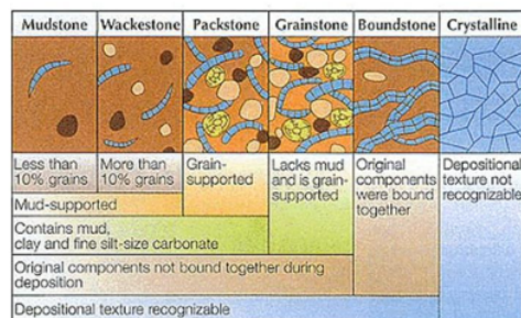
Gambar 3. Klasifikasi Batuan Karbonat (Dunham, 1962)
