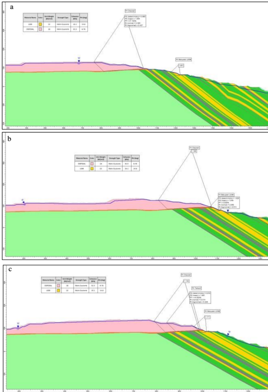
Gambar 4. Sayatan penampang lereng (a) 6X-6X', (b) 7X-7X' dan (c) 8X-8X' dengan parameter masukan nilai properties sesudah dilakukan analisis balik.
