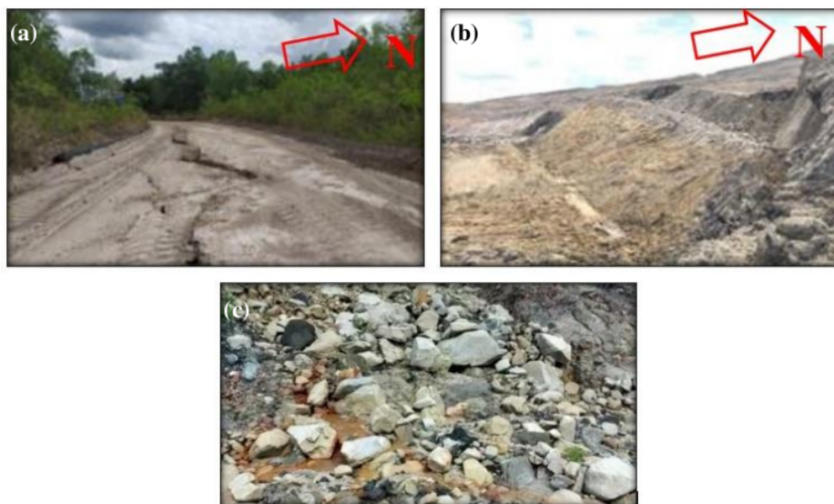
Gambar 2. Hasil pengamatan visual pada lokasi penelitian yang menjadi indikasi pergerakan lereng (a) Retakan di RL+132 timbunan, (b) Retakan di RL+86 crest Jalan Natuna dan (c) Rembesan di RL+96.
