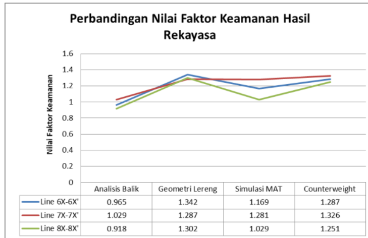
Gambar 5. Grafik Perbandingan Nilai Faktor Keamanan Hasil Rekayasa.
