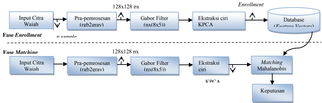
Gambar 6. Tahanan sistem identifikasi biometrika wajah
