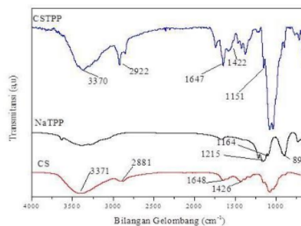
Gambar 2. Spektra FT-IR kitosan (CS), NaTPP murni dan CSTPP
