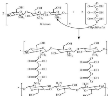
Gambar 1. Mekanisme reaksi taut silang kitosan dengan NaTPP [8]
