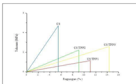
Gambar 4. Hasil uji kuat tarik membran
