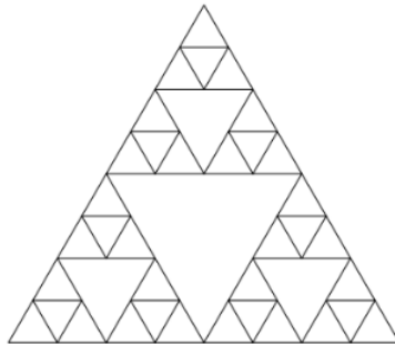
Gambar 1a. Segitiga Sierpinski iterasi ke-4
