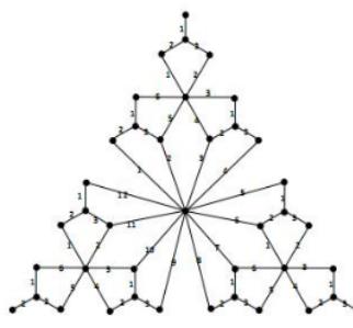
Gambar 2b. Pewarnaan sisi graf SS_4
