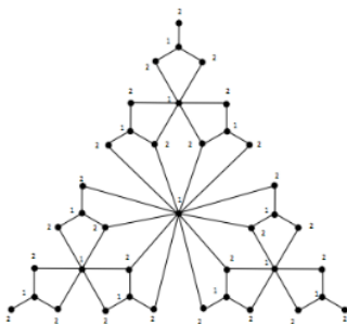
Gambar 2a. Pewarnaan titik graf SS_4
