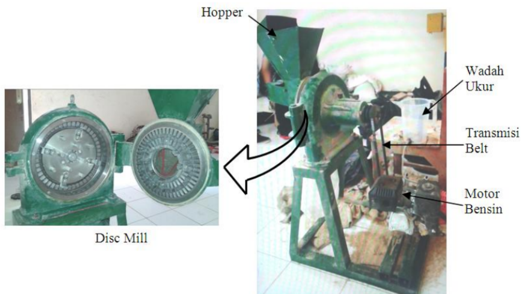
Gambar 1. Disc mill tipe FFC-XX
