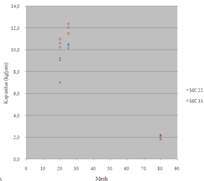
Gambar 2. Grafik Mesh versus Kapasitas (kg/jam) pada MC 22 dan MC 33
