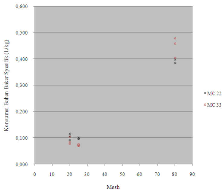
Gambar 3. Grafik Mesh versus Konsumsi Bahan Bakar Spesifik (L/kg) pada MC 22 dan MC 33
