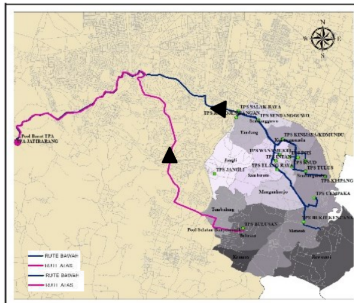
Gambar 4. Visualisasi rute pengangkutan sampah di Kecamatan Tembalang
