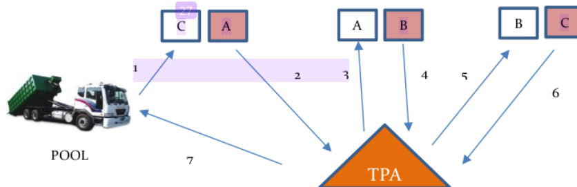
Gambar 3. Pola pengangkutan HCS Kecamatan Tembalang
