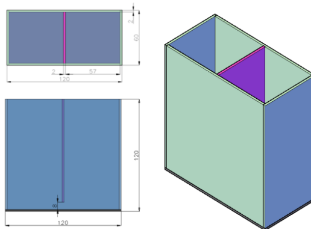
Gambar 2. Kompartemen sel elektrolisis
