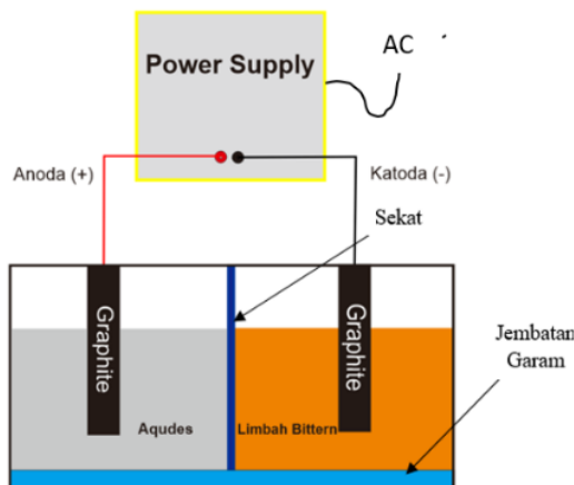
Gambar 1. Desain alat elektrolisis
