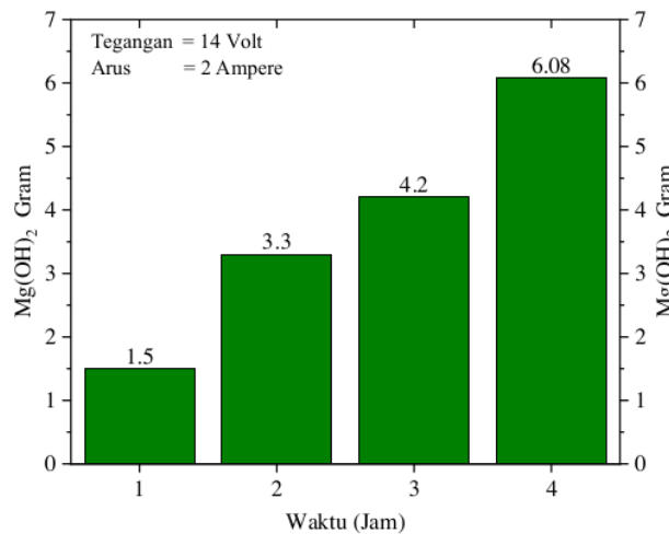
Gambar 5. Pengaruh waktu terhadap jumlah Mg(OH)_2
