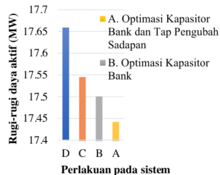
Gambar 6. Perbandingan rugi-rugi daya aktif
