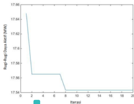
Gambar 3.4. Rugi-rugi daya aktif terkecil pada optimasi tap pengubah sadapan tanpa optimasi kapasitor bank
