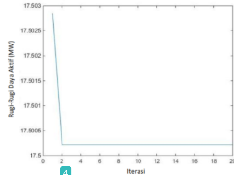
Gambar 4.4. Rugi-rugi daya aktif terkecil pada optimasi kapasitor bank tanpa optimasi tap pengubah sadapan
