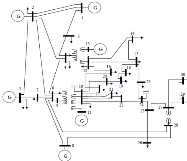
Gambar 2. Sistem IEEE 30-bus (Saadat, 1999)
