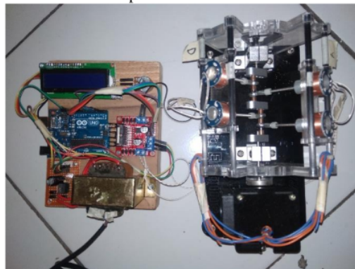
Gambar 2 Rangkaian Alat Keseluruhan
