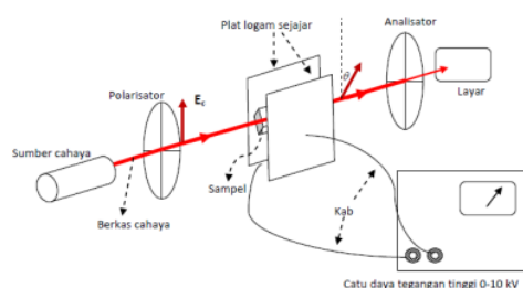
Gambar 1. Rangkaian Peralatan Polarisator [11]
