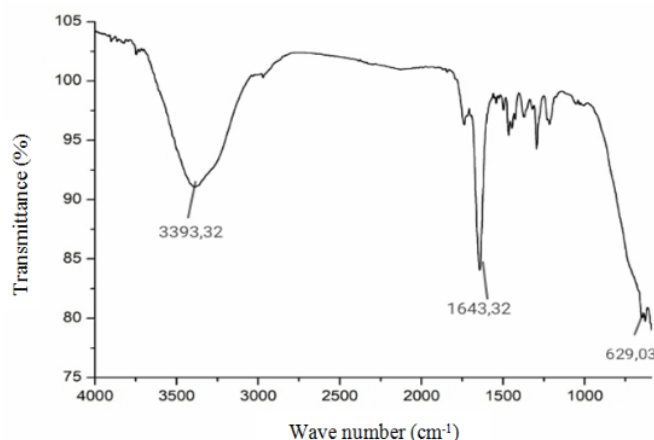
Fig. 7. SnNPs FTIR spectrum.
