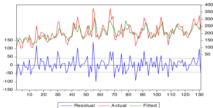
Gambar 4 Plot data produksi kentang dan prediksi dengan ARIMA([1,11],0,0)
