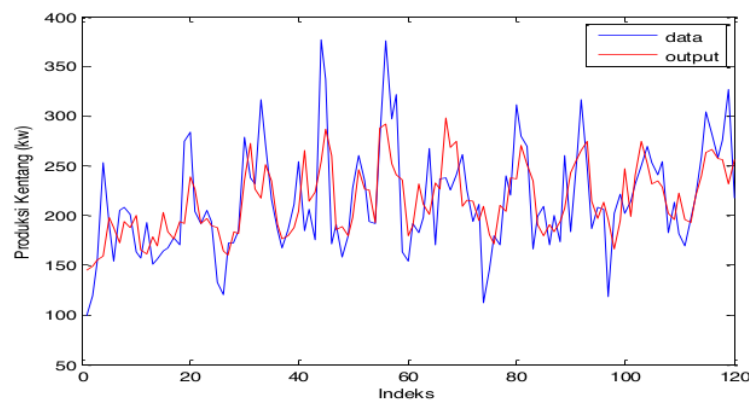
Gambar 5 Plot data in sample dan hasil prediksi produksi kentang dengan ANFIS
