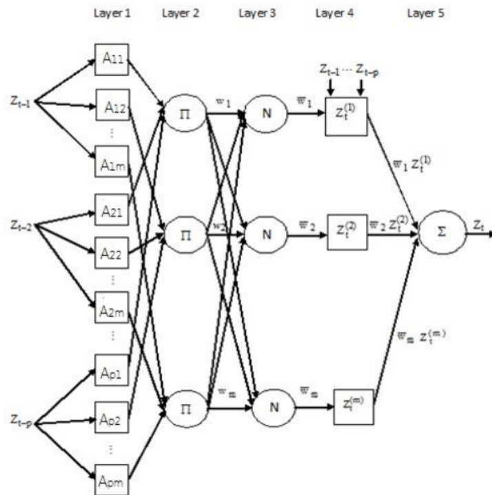
Gambar 1 Arsitektur dasar ANFIS untuk model runtun waktu.
