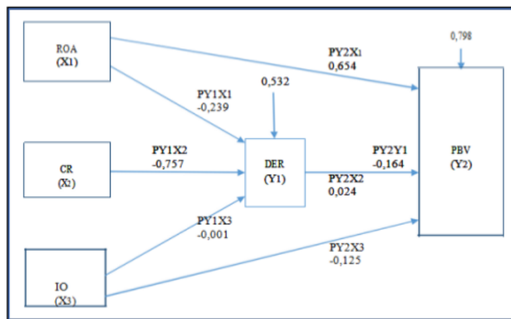
Gambar 4.42 Diagram Jalur Analisis Pengaruh Variabel ROA, CR, dan IO Terhadap PBV Secara Langsung dan Secara Tidak Langsung Melalui Variabel DER
