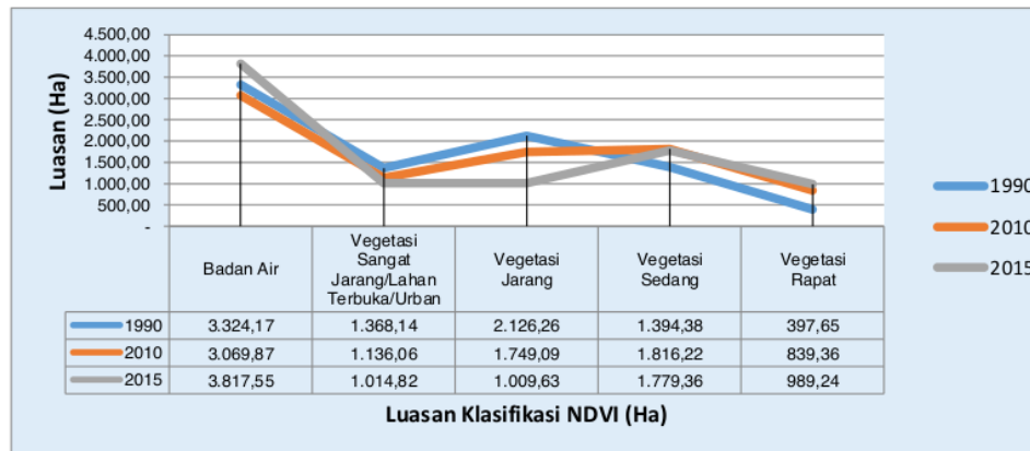
Gambar 3 Luasan Klasifikasi NDVI 1990, 2010, dan 2015
