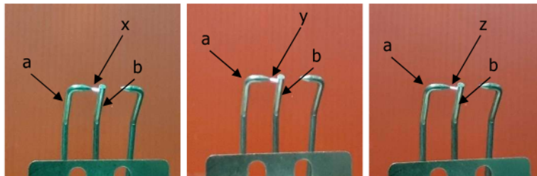
Gambar 13. Pengujian bunga api tegangan masukan 3 V, 5 V, dan 7 V (berurutan dari kiri)
