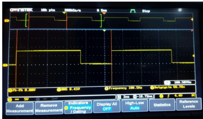
Gambar 8. Gelombang kotak 100,5 Hz duty cycle 66,78% yang dihasilkan dari proses switching pada sistem pembangkitan tegangan tinggi impuls 31,4 kV menggunakan ignition coil
