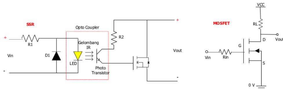
Gambar 2. SSR dan MOSFET
