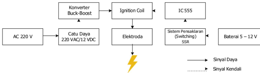
Gambar 3. Diagram blok sistem pembangkitan tegangan tinggi impuls 31,4 kV menggunakan ignition coil
