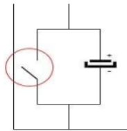
Gambar 6. Bagian rangkaian switching pada sistem pembangkitan tegangan tinggi impuls 31,4 kV menggunakan ignition coil
