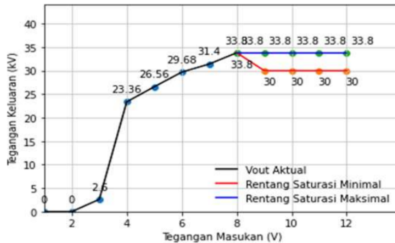
Gambar 9. Grafik korelasi tegangan masukan dan keluaran ignition coil
