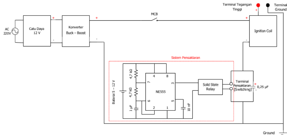
Gambar 4. Rangkaian sistem pembangkitan tegangan tinggi impuls 31,4 kV menggunakan ignition coil
