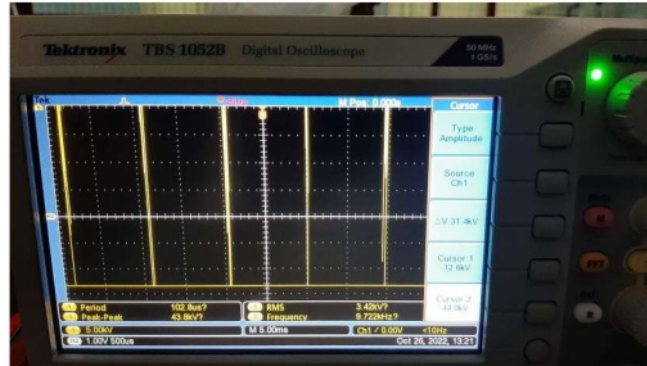
Gambar 12. Tampilan gelombang impuls dengan tegangan keluaran rata-rata 31,4 kV dan masukan 7 V
