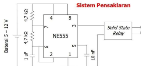
Gambar 7. Sistem pengontrol switching pada sistem pembangkitan tegangan tinggi impuls 31,4 kV menggunakan ignition coil
