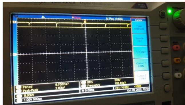
Gambar 10. Tampilan gelombang impuls dengan tegangan keluaran rata-rata 2,6 kV dan masukan 3 V
