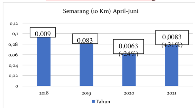
1 Gambar 3. Jumlah Kolom Atmosfer NO 2 selama April-Juni dalam Radius 10 Kilometer di Sekitar Semarang
