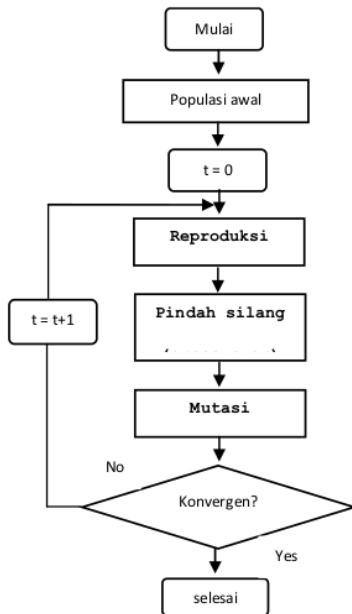
Gambar 3. Diagram alir GA.
