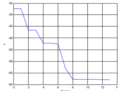
Gambar 6. Fungsi obyektif.
