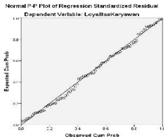
Gambar 2 Hasil Uji Normalitas Grafik Normal P-Plot
