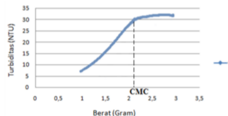
Gambar 3. Grafik nilai CMC Surfaktan Kationik Hasil Sublimasi
