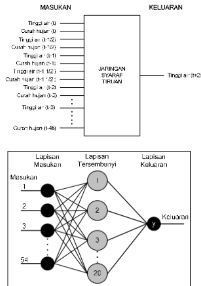
Gambar 7 Contoh struktur data masukan dan arsitektur JST untuk model satu
