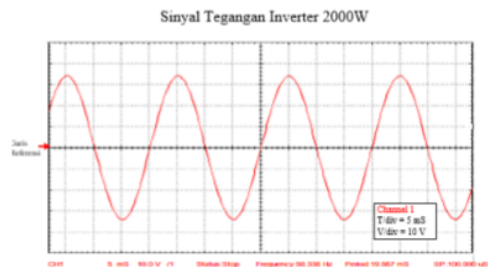
Gambar 5. sinyal tegangan output 2000 watt
