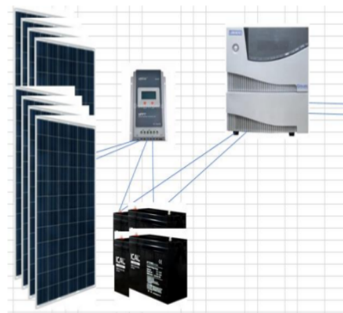
Gambar 3. konfigurasi PLTS
