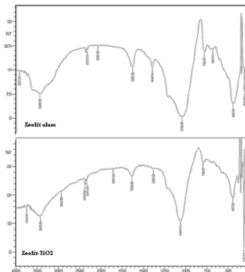
Gambar 2. Spektrogram Inframerah Zeolit aktivasi dan Zeolit-TiO 2
