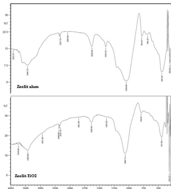
Gambar 2. Spektrogram Infra Merah Zeolit aktivasi dan Zeolit-TiO 2
