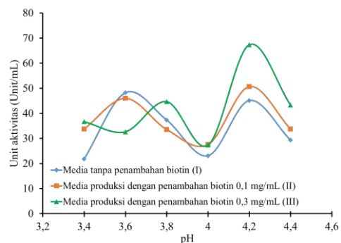
Gambar 4. Grafik pH optimum
