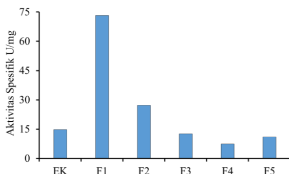
Gambar 3. Grafik aktivitas spesifik kitinase
