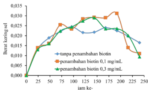
Gambar 1. Kurva Pertumbuhan Trichoderma viride FNCC6013
