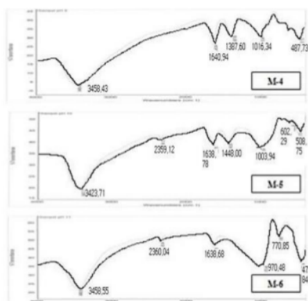
Gambar 4 Spektra FTIR Standar dan Sampel
