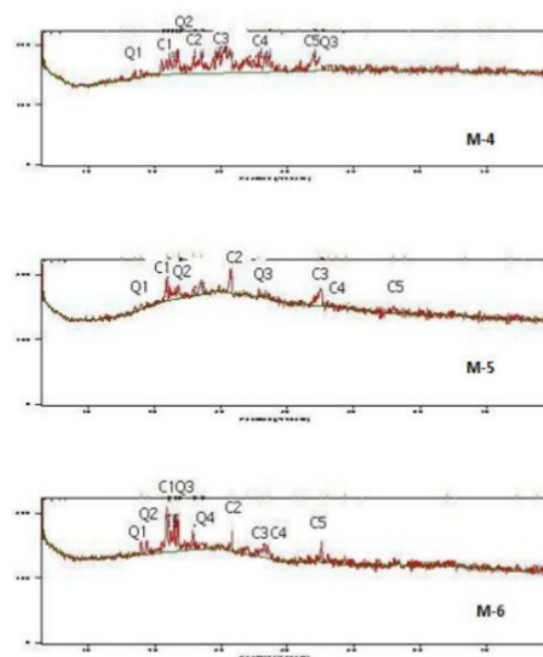
Gambar 3 Pola Difraktogram sampel M-4, M-5 dan M-6
