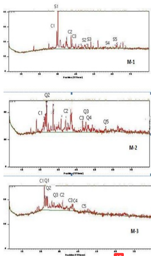
Gambar 2 Pola Difraktogram sampel M-1, M-2 dan M-3
