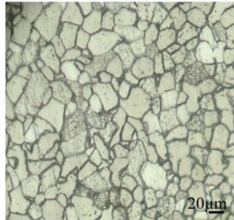
Gambar 4. Struktur Mikro Logam Induk
