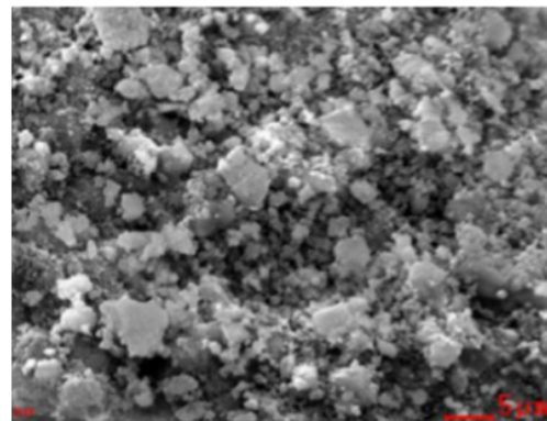
Gambar 1. Limbah geothermal setelah diproses dengan proses caustic digestion .
