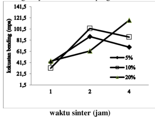
Gambar 5. Kekuatan bending komposit
