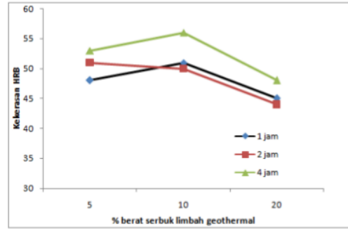
Gambar 4. Kekerasan komposit aluminium yang diperkuat serbuk limbah geothermal .
