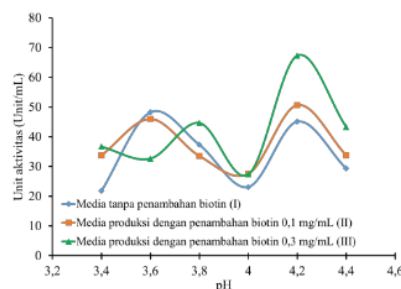
Gambar 4. Grafik pH optimum
