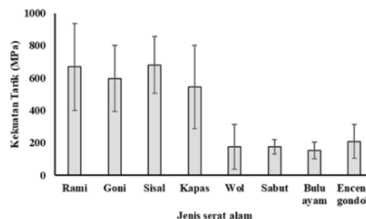
Gambar 1. Kekuatan Tarik Beberapa Serat Alam
