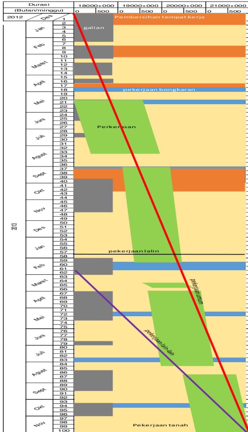
Gambar 4 Time Chainage Diagram 1m Proyek Jalan Tol Semarang-Solo Tahap I Ruas Semarang-Bawen, Seksi II Ungaran-Bawen Paket V Tinalun-Lemah Ireng (Analisis, 2018)
