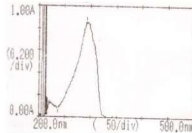
Gambar 4. kompleks [\text{Ni}(\text{acac})_2(\text{H}_2\text{O})_2] dalam pelarut aseton
