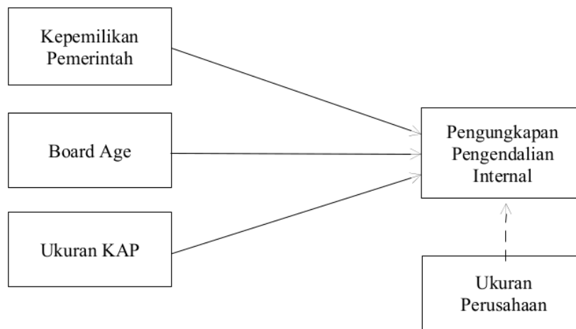
Gambar 1. Kerangka Penelitian
