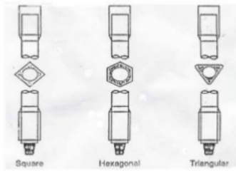
Gambar 11. Kelly
