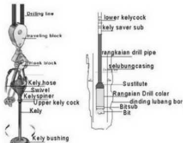
Gambar 7. Peralatan Pengeboran
