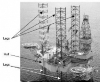
Gambar 4. Struktur Jack Up Rig
