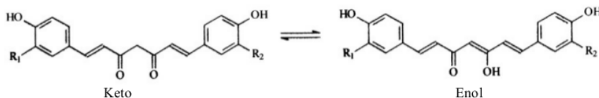
Gambar 2. Struktur keto-enol kurkuminoid
