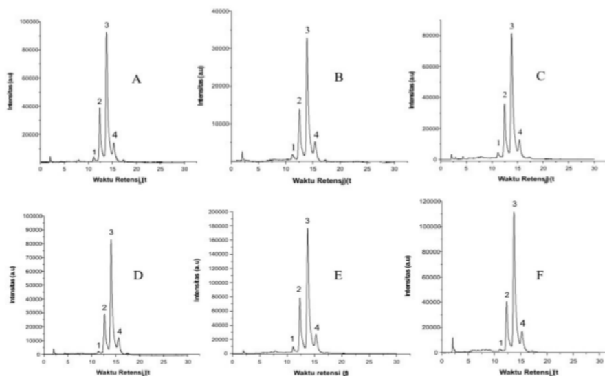
Gambar 5. Kromatogram KCKT ekstrak kurkuminoid sampel temulawak yang telah mengalami proses pengeringan, A(L1), B(L3), C(L5), D(O1), E(O3), F(O5)
