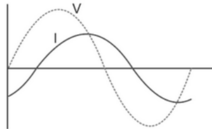
Gambar 9. Beban Induktif
