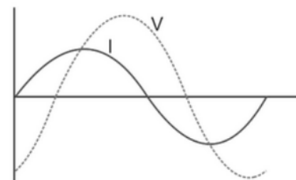
Gambar 10. Beban Kapasitif
