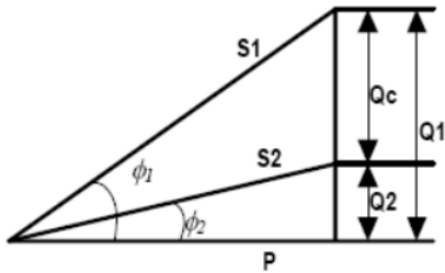
Gambar 11. Prinsip Perbaikan Faktor Daya
