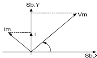
Gambar 12. Diagram Phasor V dan i Rangkaian Kapasitor
