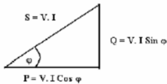
Gambar 2. Penjumlahan Trigonometri Daya Aktif, Reaktif Dan Semu
