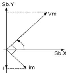
Gambar 9. Diagram Phasor V dan i Rangkaian Induktif
