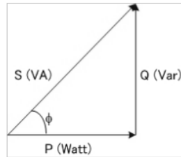
Gambar 7. Diagram Segitiga Daya
