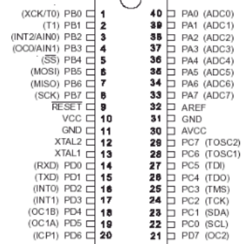
Gambar 3. Konfigurasi Pin Atmega 16
