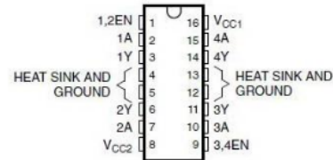
Gambar 1. Konstruksi Pin IC L293D
