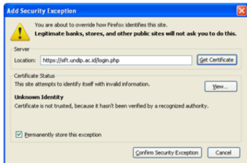
Gambar 19. Pemasangan Sertifikat secara manual
