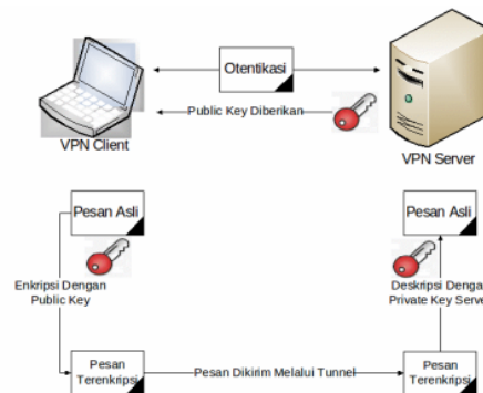
Gambar 4. Model Tunneling dengan protokol SSL
