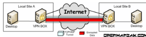
Gambar 1. Tunneling pada VPN melewati jamgan internet
