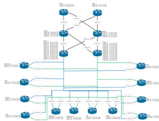
Gambar 2 topologi logikal iBGP
