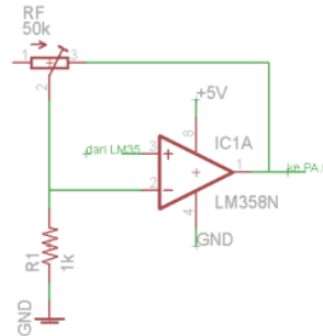
Gambar 5. Rangkaian pengkondisi sinyal
