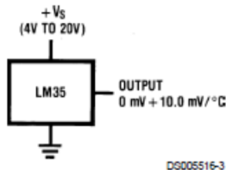
Gambar 4. Rangkaian dasar LM35
