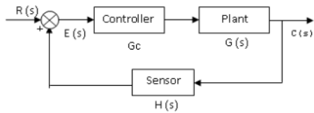
Gambar 1. Diagram blok sistem kontrol lup tertutup
