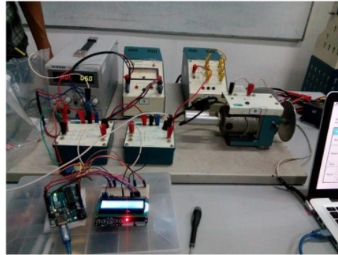
Gambar 2. Rangkaian pengujian identifikasi sistem motor DC
