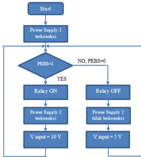
Gambar 3. Algoritma sinyal input motor DC
