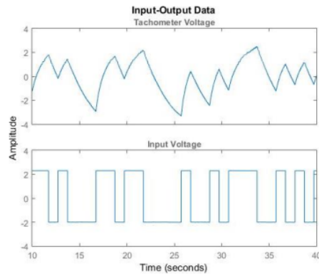
Gambar 4. Data Input-Output untuk identifikasi sistem
