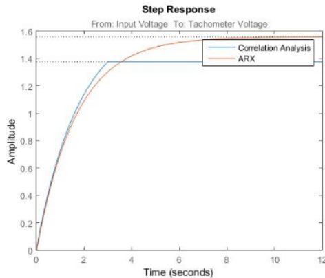
Gambar 5. Perbandingan model ARX dan Correlation Analysis terhadap masukan step
