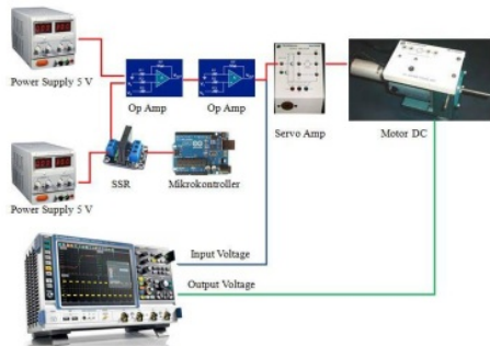
Gambar 1. Skema Eksperimen Pengambilan Data
