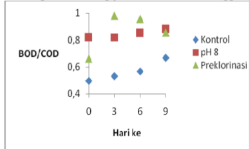
Gambar 5. Profil rasio BOD/COD limbah cair tapioka operasi start up batch ABR
