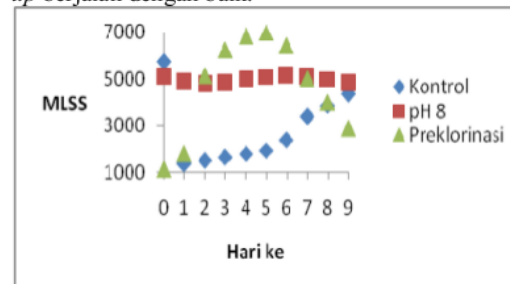
Gambar 2. Profil MLSS limbah cair tapioka operasi Start Up Batch ABR
